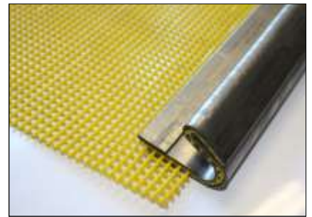
PU-Flex med 3 mm hål och 1,5 mm PU-belagd tråd.
